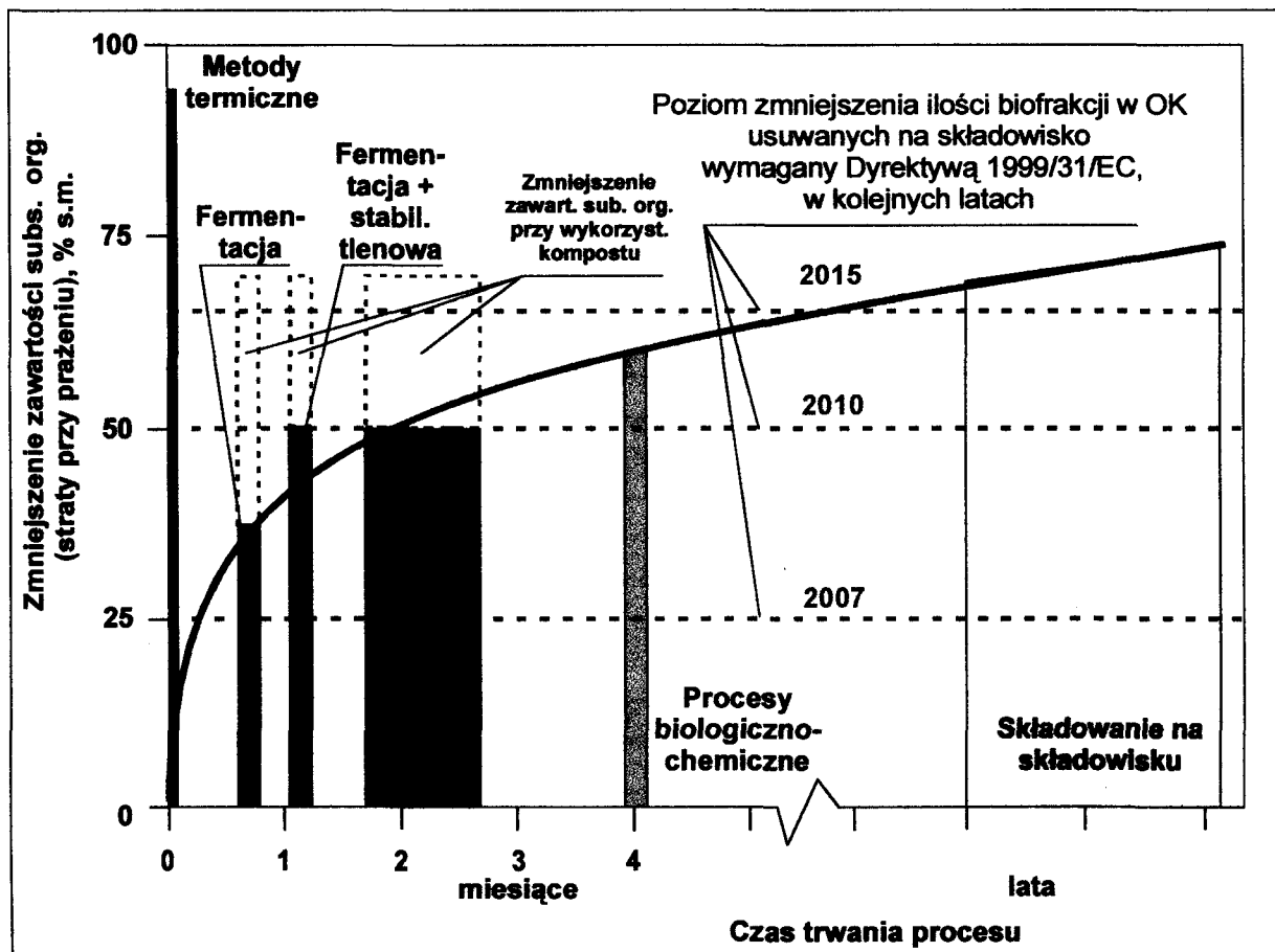
Rys 6. Stopień zmniejszania ilości substancji organicznych w odpadach komunalnych w różnych metodach ich unieszkodliwiania oraz czasie trwania procesów
